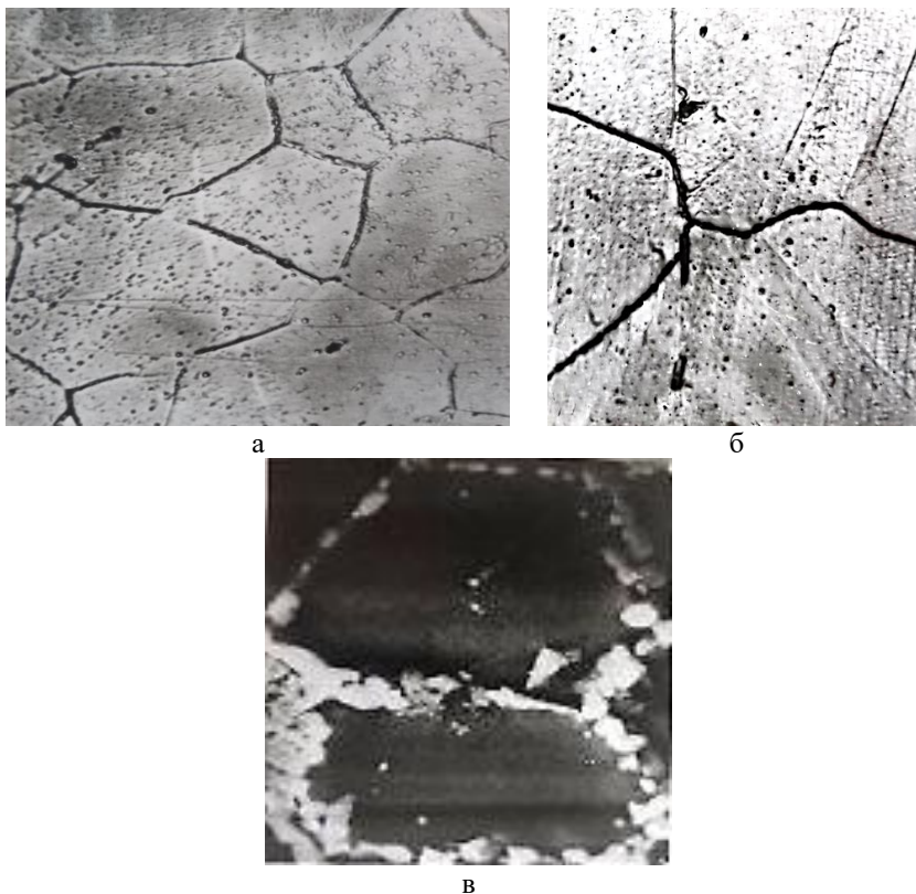
Рисунок 5 – Локальні виділення часток другої фази. а – СЕМ, x1000, б – РЕМ, x1300, в – x2500
