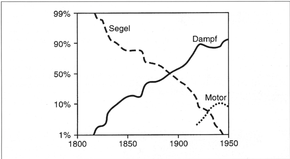
Abb. 1 Anteil der Dampf-, Segel- und Motorschifffahrt an der Handelstonnage der USA (in einer logarithmischen Skala) nach MARCHETTI (1988). Es gibt eine Initiation (siehe Abb. 2) ökonomisch erfolgreicher Dampfschifffahrt zu Beginn des 19. Jahrhunderts, der eine langsame, zunächst annähernd exponentielle Ausbreitung auf dem Schifffahrtsmarkt folgte. Man erkennt die formale Analogie der Ausbreitung technischer Innovation zur Populationsdynamik biologischer Evolution.
