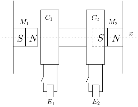
Fig. 47: Generator
