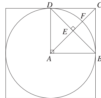
Fig. 42: Internal tangent circle
