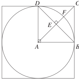
Fig. 43: Internal tangent circle
