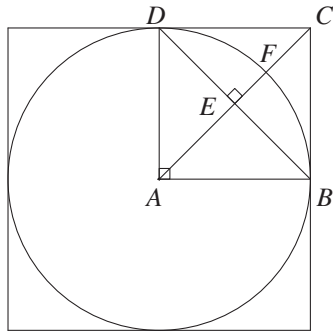
Fig. 30: Internal tangent circle
