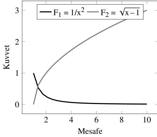
Fig. 6: Yukarıda belirtilen hesaplamalara göre olası Galaksi dönüş eğrisi Burada F_1 klasik Newton hesabıdır ve mesafenin karesiyle ilişkilidir kuvvet ve dolayısı ile hız. F_1 kuvveti ile oluşan dönüş eğrisinin grafikteki gibi olması beklenir. F_2 ise denklem (13) üzerinden AO=1 için değişen AD ve OD değerleriyle yazılmış yeni denklem (13) olan F = \sqrt{x-1}/x^2 kuvveti ve F_1 yani Newton hesabına göre oluşan kuvvetin oranıdır. Oran ölçüsünde kuvvet ve dolayısı ile hız kaynaklı oluşan dönüş eğrisinde grafikteki gibi artış görülür Newton hesabına nispeten.
