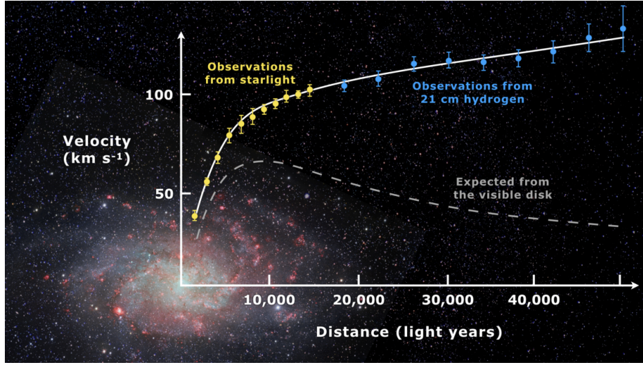
Fig. 7: Wikipedia'dan sarmal gökada Messier 33'ün dönme eğrisi. Fig. 6 ile benzerlik aşıkardır.
