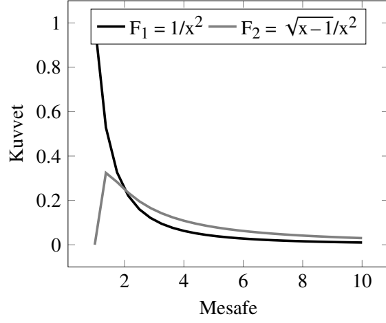
Fig. 5: Yukarıda belirtilen hesaplamalara göre kuvvet değişimleri Burada F_1 klasik Newton hesabıdır. F_1 kuvveti ile oluşan kuvvet eğrisinin grafikteki gibi olması beklenir. F_2 ise denklem (13) üzerinden AO=1 için değişen AD ve OD değerleriyle yazılmış yeni denklem (13) olan F = \sqrt{x-1}/x^2 kuvvetidir. Global minimum ve maksimum noktaları vardır ve bu durum, kuantum mekaniği; özellikle nükleer fizik için önemlidir. Mesafe küçüldükçe kuvvet her zaman artmaz.
