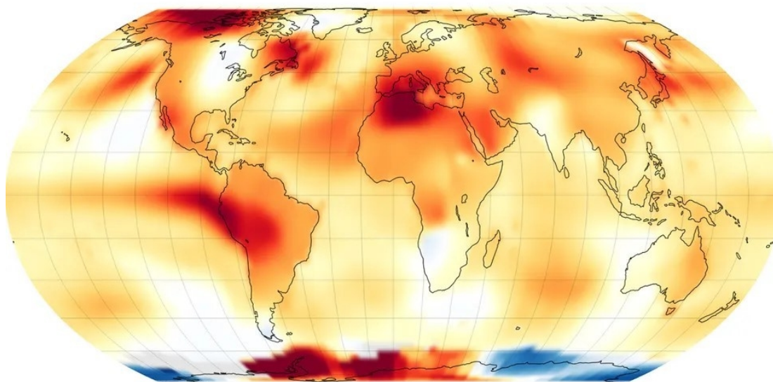
Bản đồ phân bố nhiệt độ tháng 7/2023 (dữ liệu NASA dẫn theo [2])
