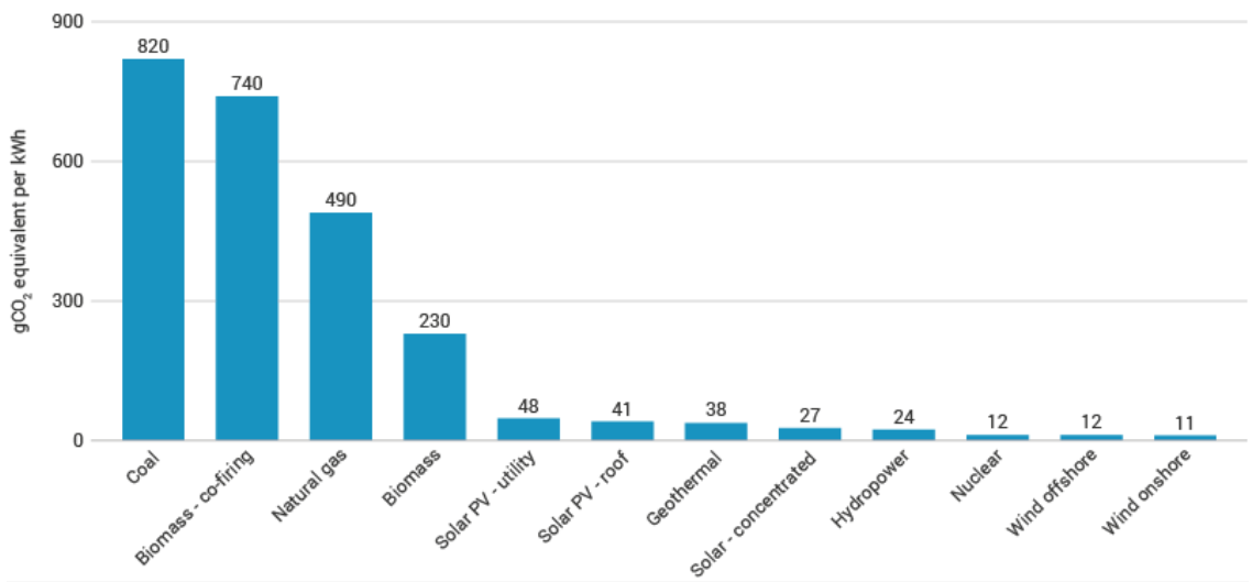
Lượng phát thải trung bình tương đương lượng carbon dioxide trong vòng đời của các máy phát điện khác nhau (Nguồn: IPCC)
