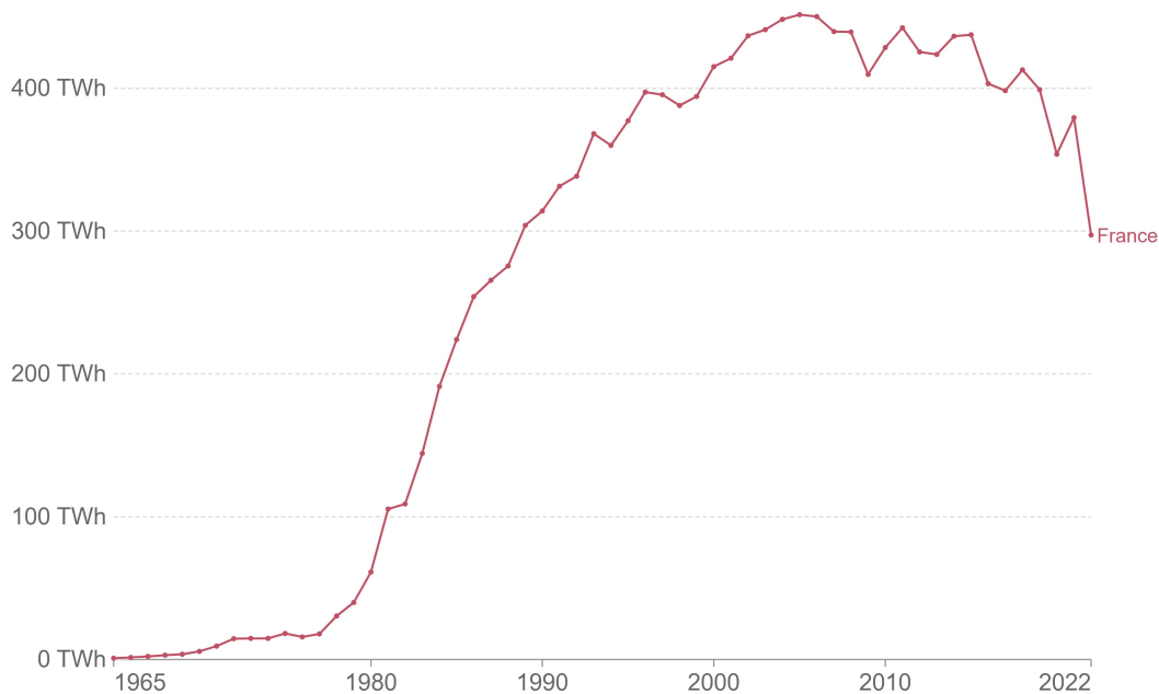
Sử dụng điện hạt nhân tại Pháp tính đến năm 2022 (nguồn ourworlddata)
