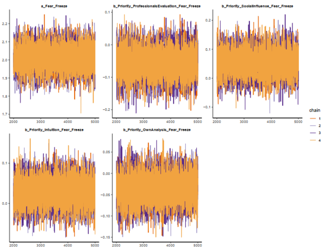
Hình 4: Biểu đồ truy vết Mô hình 1
