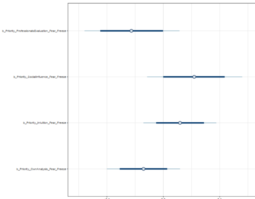
Hình 5: Phân phối hậu nghiệm của hệ số Mô hình 1
