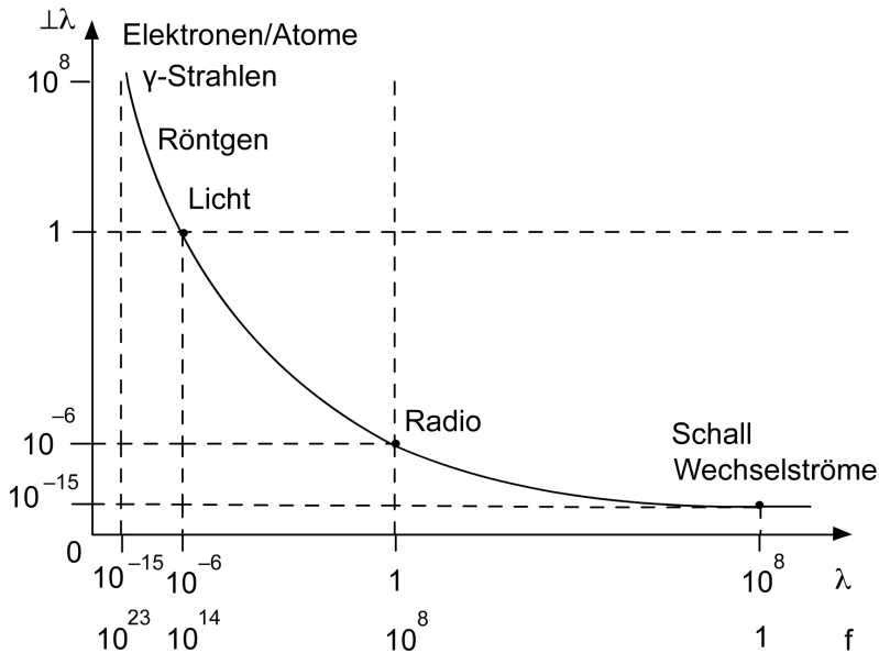
Abb. 8 Das geometrische Wellen-Spektrum. Die Verhältnisse zwischen den Wellenklassen sind in einem Diagramm zusammengefasst, und beziehen sich auf die Positionen, wo die Maßgrößen \lambda und \frac{1}{\lambda} jeweils den Wert von 1 annehmen. Das Spektrum bekommt damit die Symmetrieachsen, die den Raum dieses Diagramms unterteilen, was bei einer traditionellen Darstellung nicht zum Vorschein kommt.
