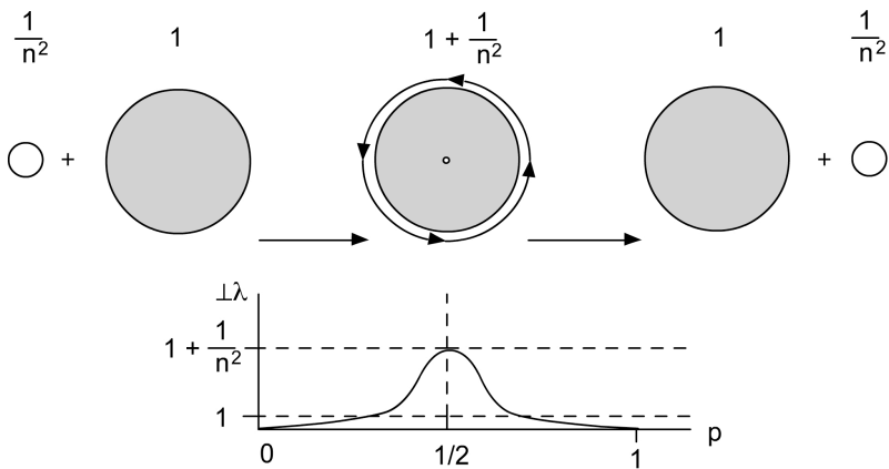
Abb. 7 Eine verallgemeinerte Darstellung der Periodizität. Während das Atom eine elementare Quantität aufnimmt (Absorption), dehnt es aus (Ausdehnung wenn n > 1 , Unterteilung wenn n = 1 ). Bei \Delta\lambda = 1 befindet
