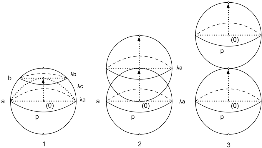
Abb. 3 Hypothetische Ereignisse zur Veranschaulichung von Flächenverteilung innerhalb einer Sphäre. Während die Fläche a sich immer mehr in die Richtung eines Pols bewegt, und anschließend aus dem gemeinsamen Raum austritt und verselbständigt, ändert sich das Verhältnis zwischen \lambda und p .
