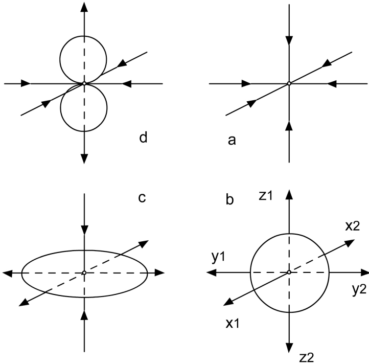
Abb. 4 Koordinatensysteme in einem multifocalen Universum. Jeder Punkt des Raumes stellt eine singuläre Potenz dar (a entspricht etwa den Knotenpunkten einer stehenden Welle), die verschiedene Konformationen annehmen kann: Aus dem Null-Punkt kann infolge der Ausdehnung eine Form entstehen (c und b entsprechen den 2-D- und 3-D-Flächen); die Ausdehnung weicht der Unterteilung (d). Die Superposition des Raumes entsteht infolge überlappender und aufsteigender Kreise der Wechselwirkungen, wo es keine Unterbrechung zwischen Mikro- und Makrozuständen gibt. Die Zustandsdauer wird als Zeiteinheit definiert, die Zeit erscheint als eine permanente Größe, die aus einzelnen Zuständen
