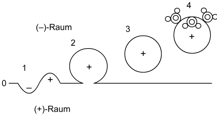
Abb. 2 Elementare Ereignisse an der Grenze zwischen 2 Phasen infolge der Vakuolierung (Nukleierung) des Raumes. Eine Membrane teilt den Raum in zwei Hälften, die sich als (+)- und (-)-Räume in Bezug aufeinander bzw. in Bezug auf die Grenze definieren. Die Grenze hat Dimension 2D, die entstehenden Formen weisen eine 2/3-D Struktur auf. Eine symmetrische Schwingung induziert die Raumpolarisation (1). Die nachfolgende Unterteilung des Raumes geht über die Kompartimentbildung (2-3), und bewirkt weitere Differenzierung, die sich selbst erhält (4).
