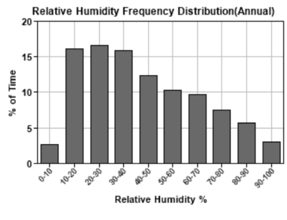
شکل ۴-۴۴- توزیع فرکانس رطوبت نسبی.
