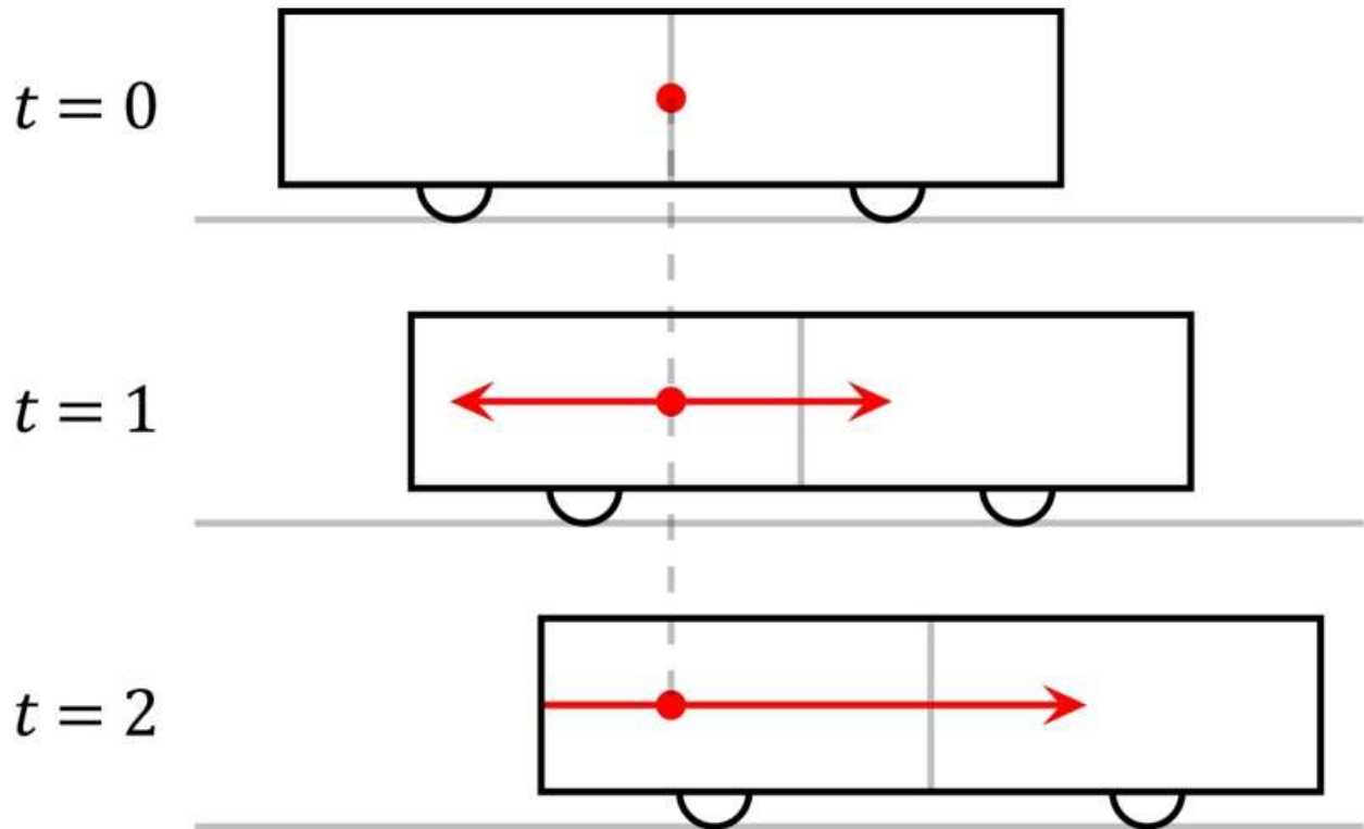
(Cadrul de referință al unui observator care se află pe calea ferată (construcția lungimii nu este prezentată). https://en.wikipedia.org/wiki/File:Traincar_Relativity2.svg )
