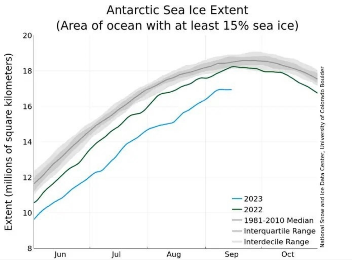
Biểu đồ thể hiện phạm vi băng biển ở Nam Cực trong giai đoạn 1981-2010 và các năm 2022 và 2023 [1]
